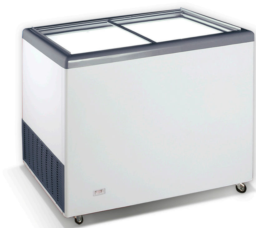
EKTOR 36 SGL 1184 x 644 x 895 356lt
